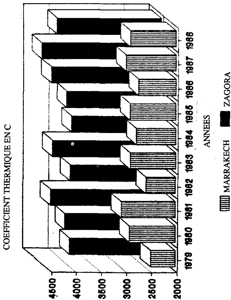
Fig 2 : Comparaison du coefficient thermique de Marrakech et Zagora (méthode de SWINGLE)
