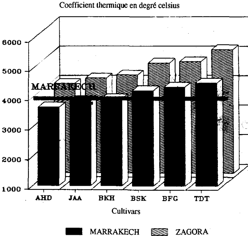
Fig 4 : Comparaison du coefficient thermique de Marrakech par rapport aux cultivars précoces de Zagora .
