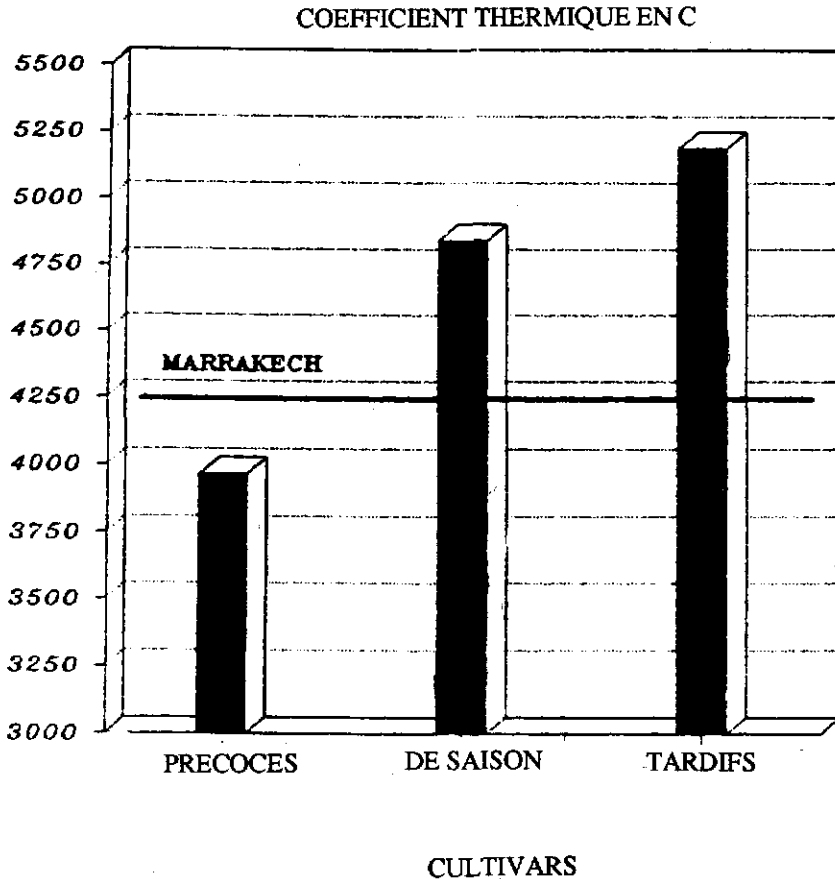
Fig 3 : Comparaison du coefficient thermique de Marrakech par rapport aux cultivars de Zagora .
